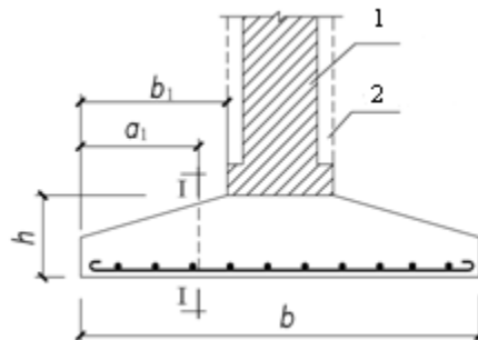
图 8.2.14 墙下条形基础的计算示意图
