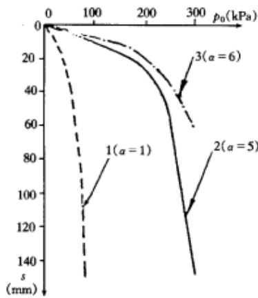
图 5 现场载荷试验 p-s 曲线
