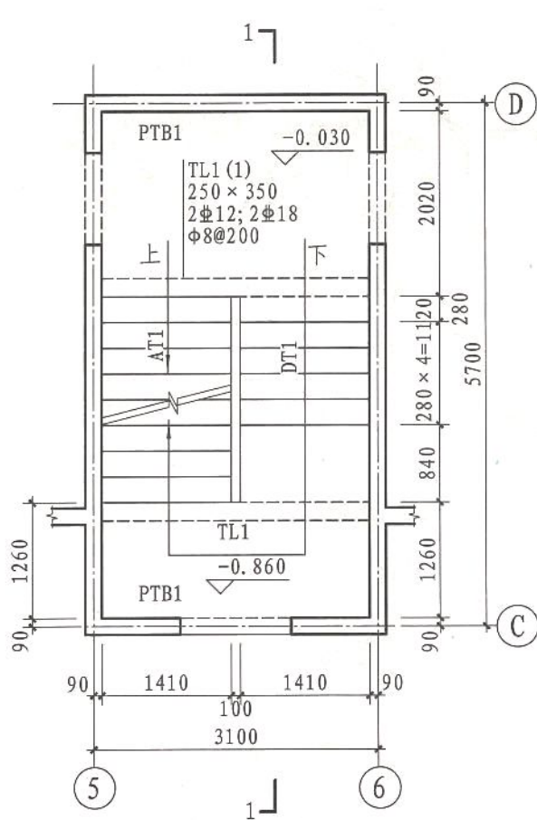
标高-0.860~标高-0.030楼梯平面图
