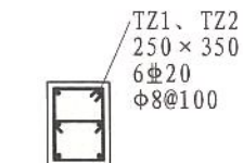
TZ1、TZ2
