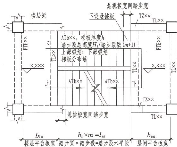
ATb型注写方式 标高x. xxx~标高x. xxx楼梯平面图
