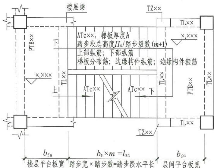
ATc型注写方式1 标高x.XXX~标高x.XXX楼梯平面图 (楼梯休息平台与主体结构整体连接)
