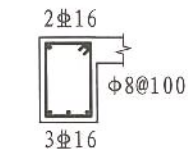
TL2 280 × 400
