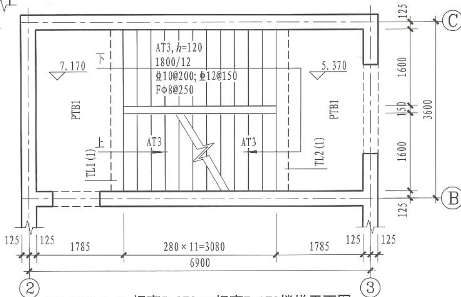
图2 设计示例 标高5.370~标高7.170 楼梯平面图
