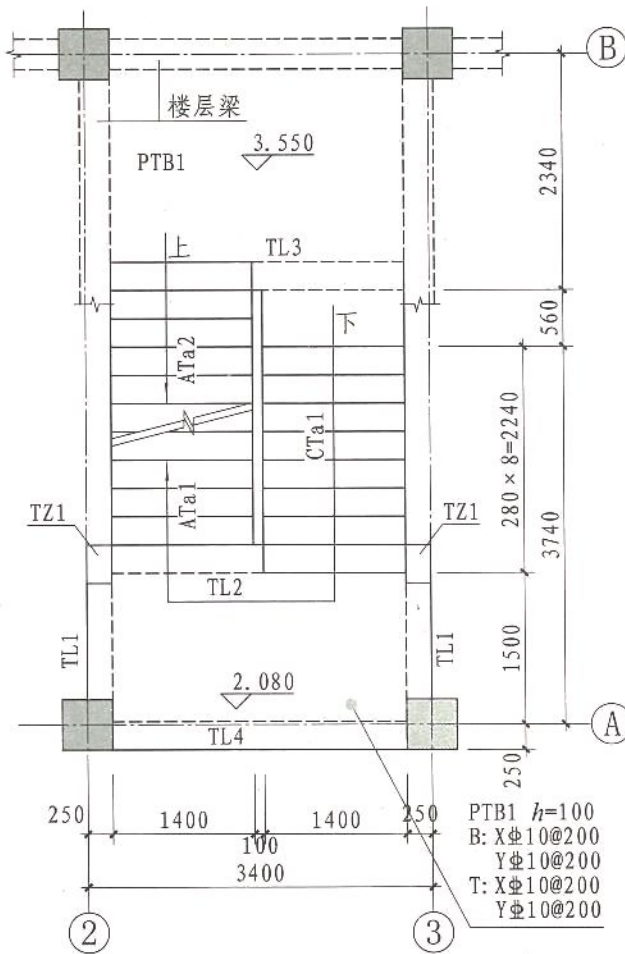
标高2.080~标高3.550楼梯平面图
