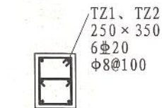
TZ1、TZ2
