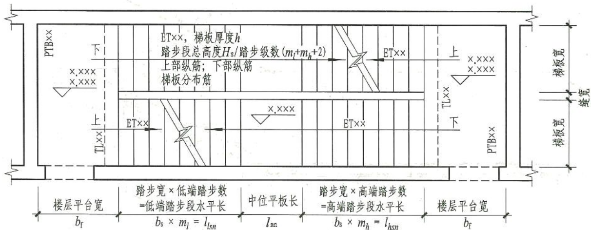
图1 注写方式 标高x.xxx~标高x.xxx楼梯平面图
