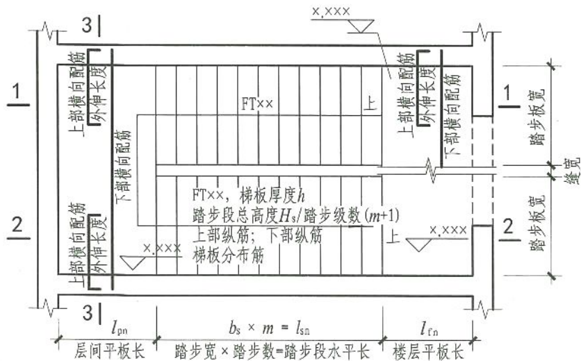
图1 注写方式1 标高x.xxx~标高x.xxx楼梯平面图
