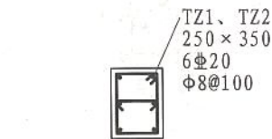
TZ1、TZ2
