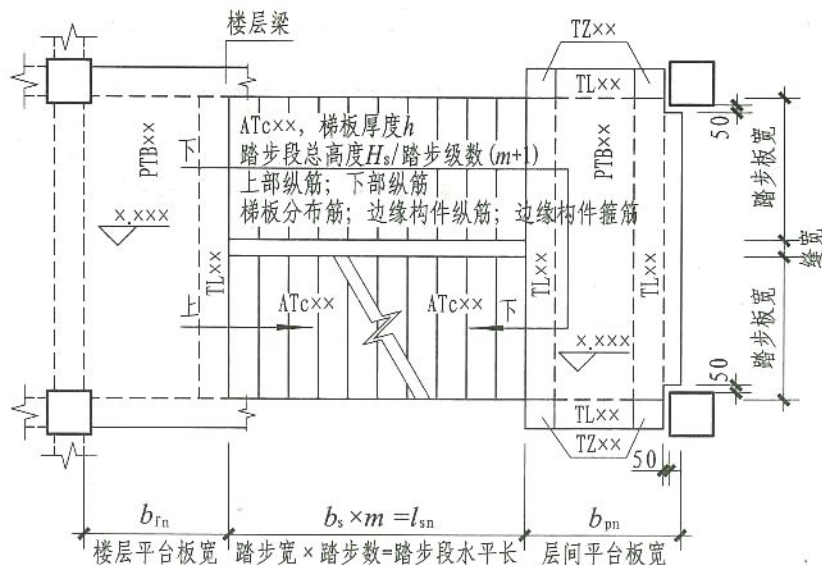
ATc型注写方式2 标高x.XXX~标高x.XXX楼梯平面图 (楼梯休息平台与主体结构脱离连接)
