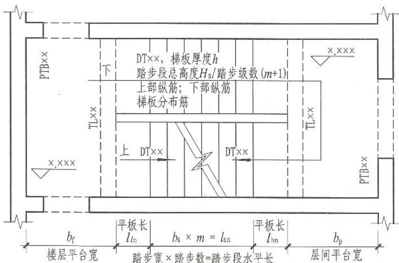
图1 注写方式 标高x.xxx~标高x.xxx楼梯平面图
