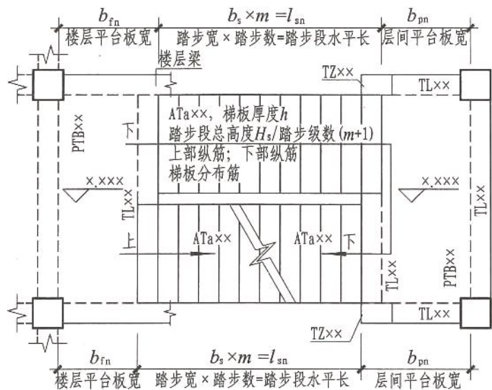
ATa型注写方式 标高x. xxx~标高x. xxx楼梯平面图
