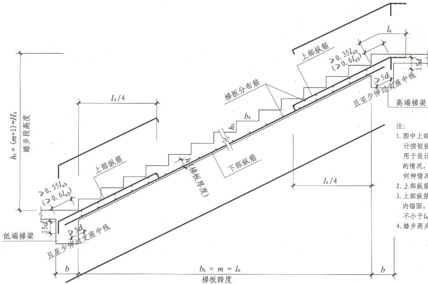
AT型楼梯板配筋构造
