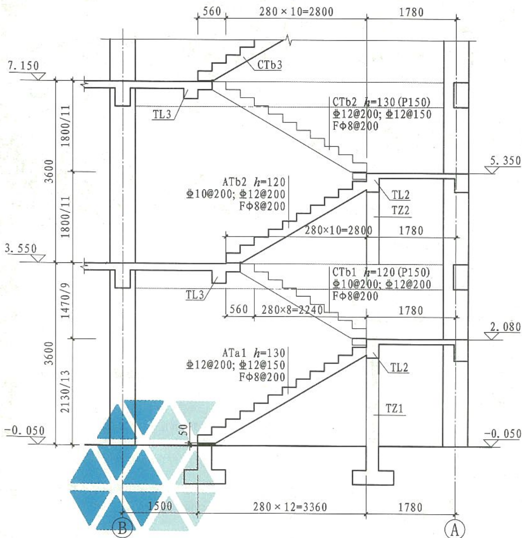
楼梯剖面图
