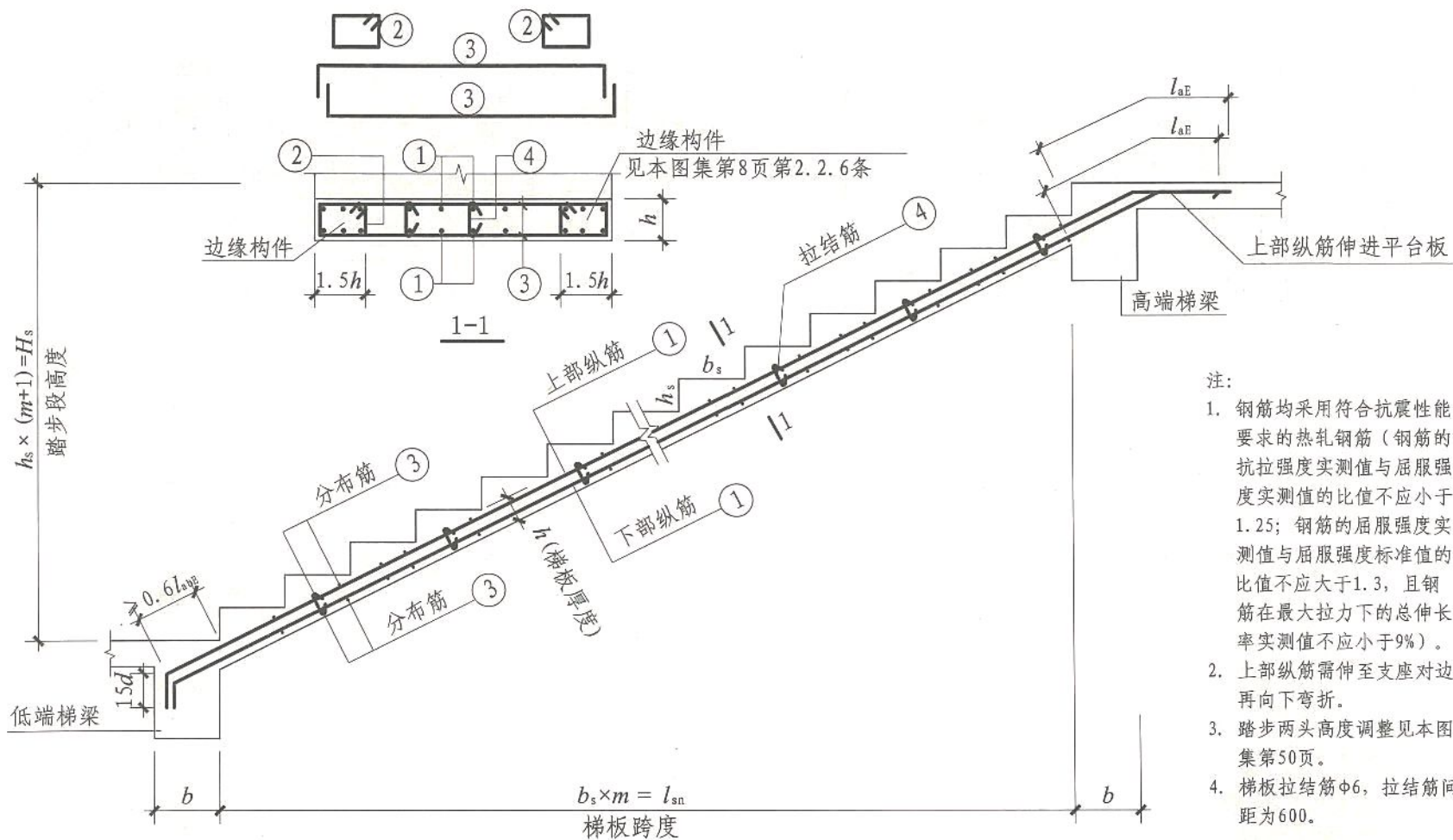
ATc型楼梯板配筋构造
