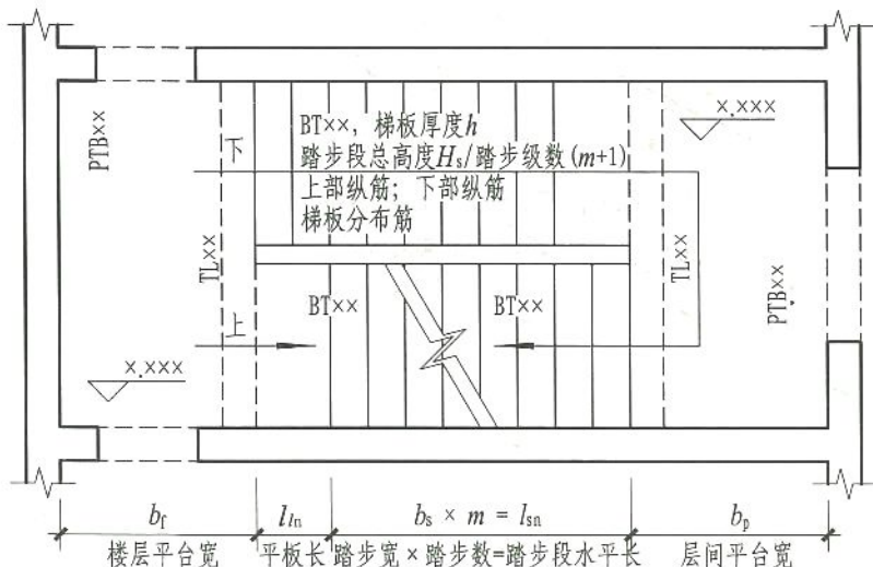
图1 注写方式 标高x.xxx~标高x.xxx楼梯平面图
