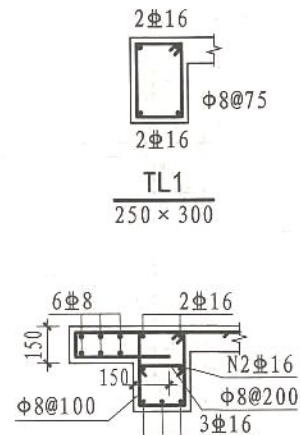
(a) 用于有挑板处
